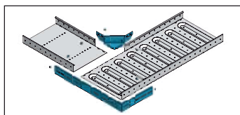
Hoekstuk t.e.m. 600 met koppelstuk 896.00.00
