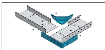
Hoekstuk t.e.m. 330 met koppelstuk 894.00.00
