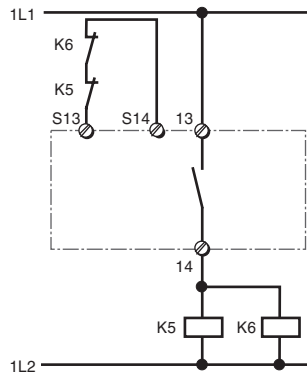
Fig. 8: Anschlussbeispiel für externe Schütze, einkanalig, automatischer Start/ Connection example for external contactors/ relays, single-channel, automatic reset/ Branchement contacteurs externes, commande par 1 canal, validation automatique
