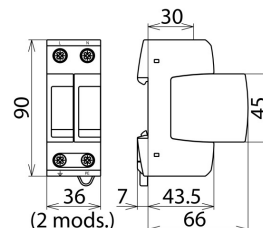
Dimensions DG M TT 2P 275
