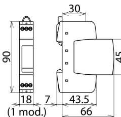
Dimensions DR M 2P 255
