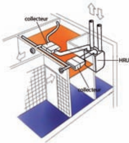
1. Montage des collecteurs d'air en faux-plafond.
