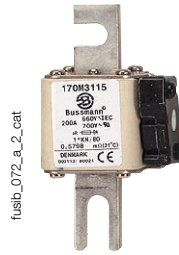
Zekering type K/50/80/110 Met inkeping
