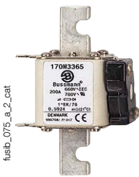
Zekering type K/76/86/91 Met inkeping
