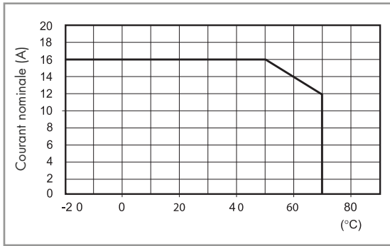
L 97 - Courant nominal en fonction de la température ambiante (pour ensemble monté relais 46.61 et support 97.01)
