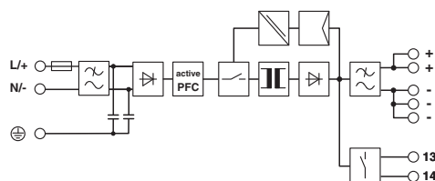
blokschema
