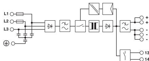
blokschema
