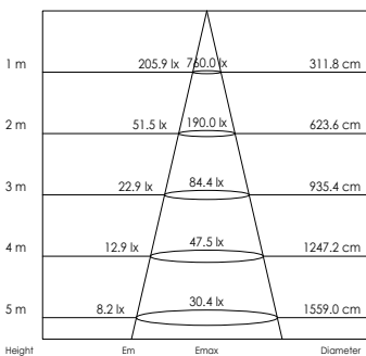
DIAGRAMMEN GEBASEERD OP 40004250 (Ø 215 MM / 3000K / 30W) DIAGRAMMES BASÉS SUR 40004250 (Ø 215 MM / 3000K / 30W)
