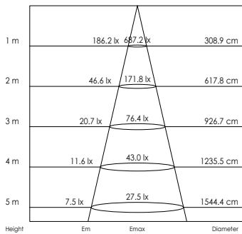
DIAGRAMMEN GEBASEERD OP 40004310 (215X215 MM / 3000K / 30W) DIAGRAMMES BASÉS SUR 40004310 (215X215 MM / 3000K / 30W)
