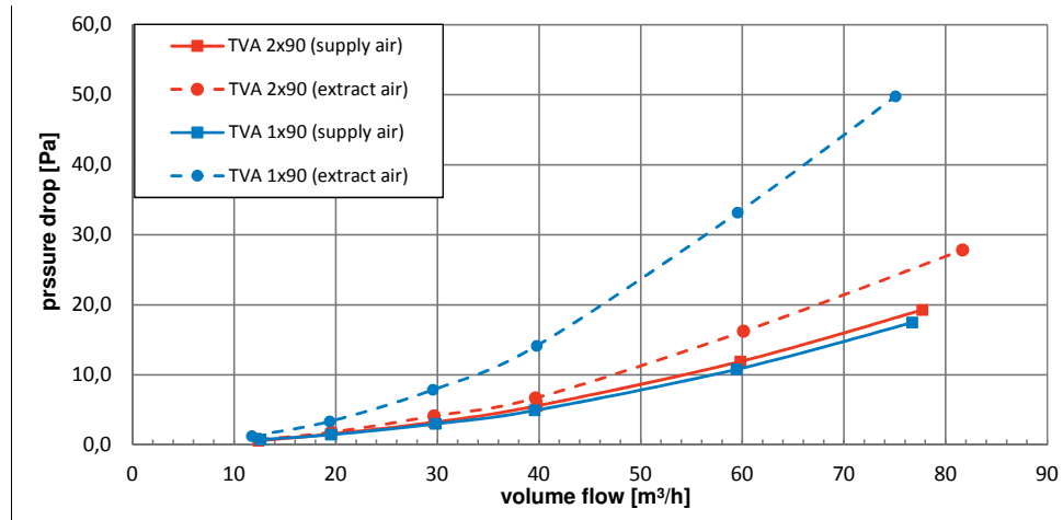
Graphique pertes de pression Plénums TVA-P 90° DN125/1xDN90 et DN125/2xDN90
