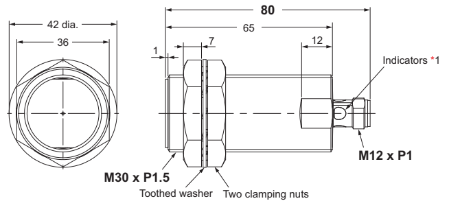
E2E-X□L30-M1
