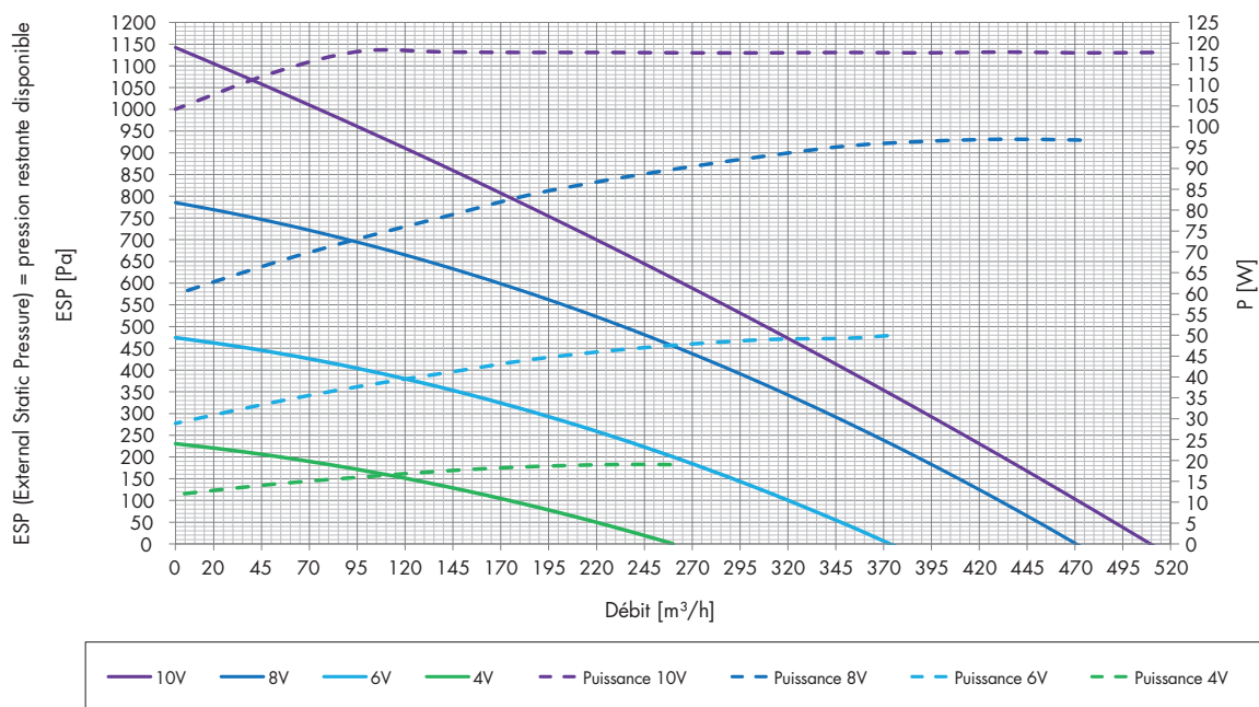
Courbes de ventilateur Endura Delta 450 pression en fonction de débit
